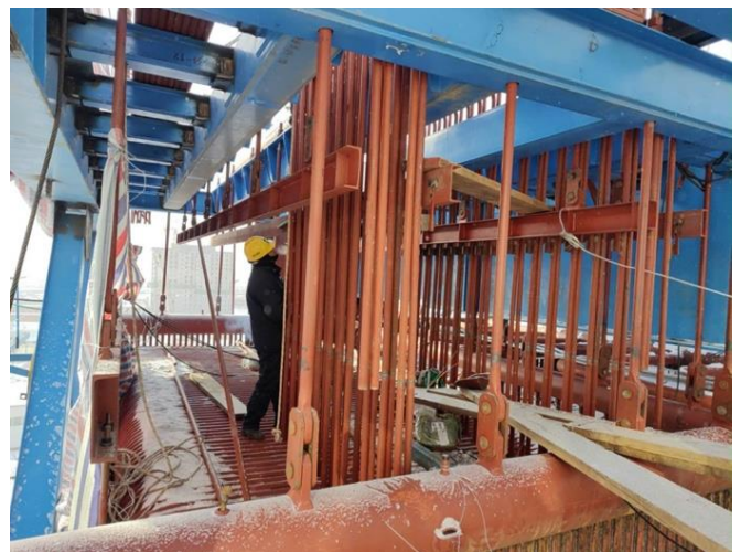
Халуун усны гаралтын коллекторын хоолой угсралт
