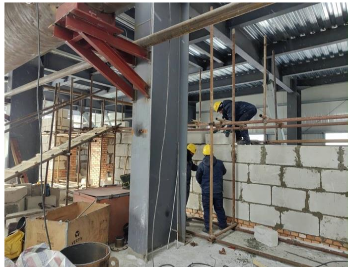
8м давхрын тоосгон ханын өрлөг шавардлага
