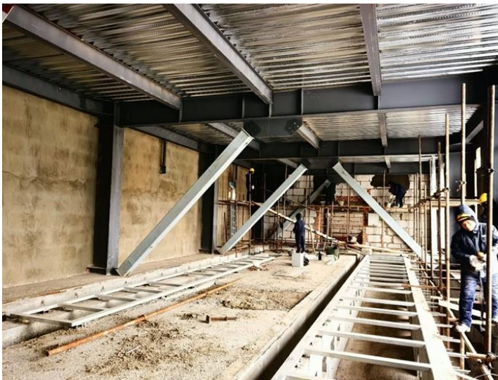
Цахилгаан түгээх өрөөний доторх ханын
